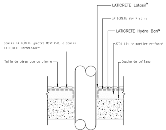
Détail 6 ES-WP300
