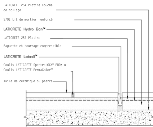
Détail 5 ES-EJ10
