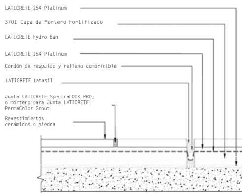
Detalle constructivo 5 ES-EJ10
