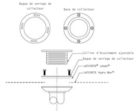
Détail 2 ES-WP302
